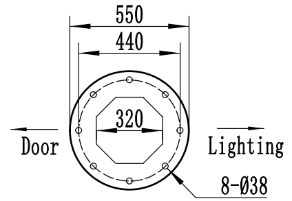
Baseplate
